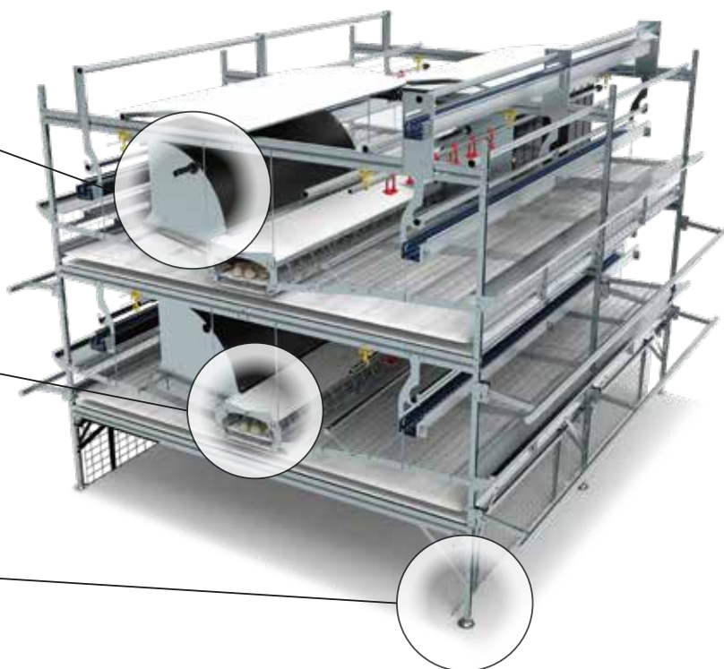
Nastro raccolta uova centrale su tutti i piani larghezza 290 mm
